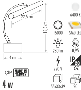
CT-5206 FLAMİNGO LEDLİ APLİK
