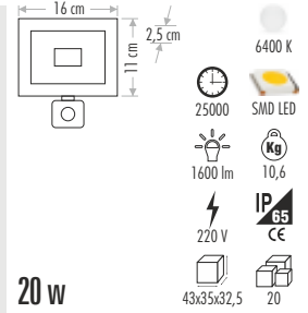
CT-4652 SENSÖRLÜ SLİM LED PROJEKTÖR 155,00 ₺
