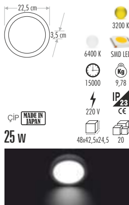
CT-5272 SIVA ÜSTÜ LED ARMATÜR
