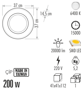
CT-4687 200 watt PENDANTE 1.000,00 ₺
