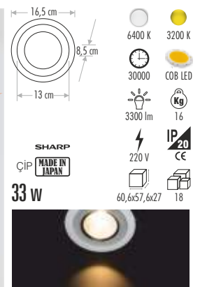
CT-5352 5" CLASS LED ARMATÜR YÜKSEK TAVAN 300,00 ₺
