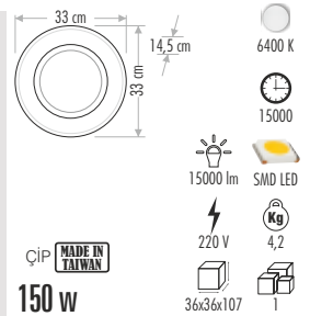
CT-4686 150 watt PENDANTE 820,00 ₺
