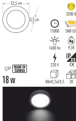
CT-5234 SIVA ÜSTÜ LED ARMATÜR
