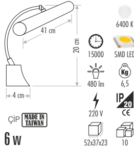
CT-5207 PELİKAN LEDLİ APLİK
