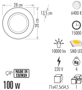
CT-4685 100 watt PENDANTE 550,00 ₺
