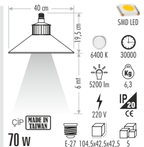
CT-4628 70 watt PENDANTE 270,00 ₺
