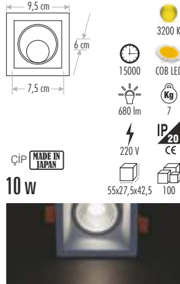
CT-5161 2" MERCAN BEYAZ GÖVDE 35,00 ₺
