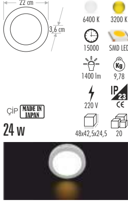
CT-5272 SIVA ÜSTÜ LED ARMATÜR
