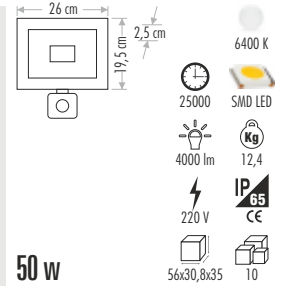
CT-4654 SENSÖRLÜ SLİM LED PROJEKTÖR 250,00 ₺
