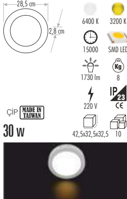
CT-5274 SIVA ÜSTÜ LED ARMATÜR
