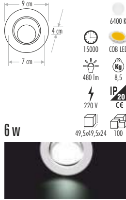
CT-5202 2" AKİK BEYAZ GÖVDE 15,00 ₺
