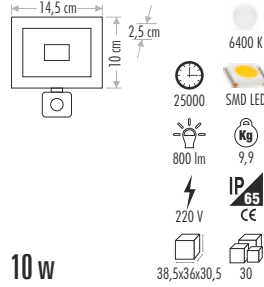
CT-4651 SENSÖRLÜ SLİM LED PROJEKTÖR 135,00 ₺
