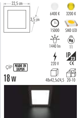
CT-5234 S DAMLA LED ARMATÜR SIVA ÜSTÜ
