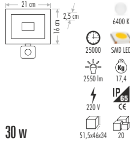
CT-4653 SENSÖRLÜ SLİM LED PROJEKTÖR 200,00 ₺
